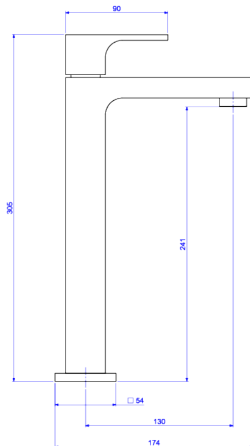
Desenho Técnico
