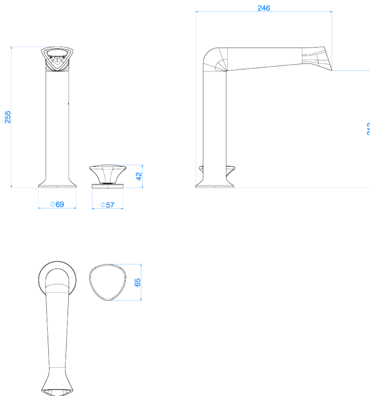
Desenho Técnico
