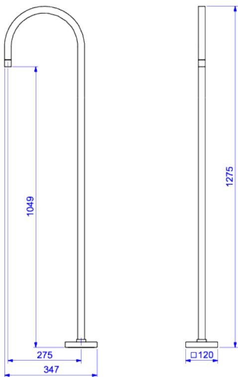
Desenho Técnico
